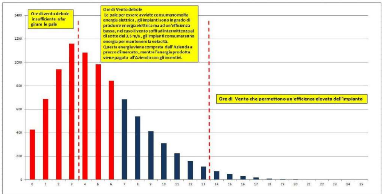
Fig. 4: Ore annuali di vento, in funzione della velocità (m/s) più o meno utili all'elettrogenazione:
